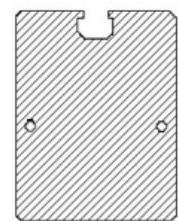
8mm Montagennut
