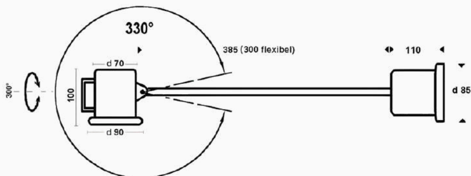
275.90.02 (mit Magnetfuß)
