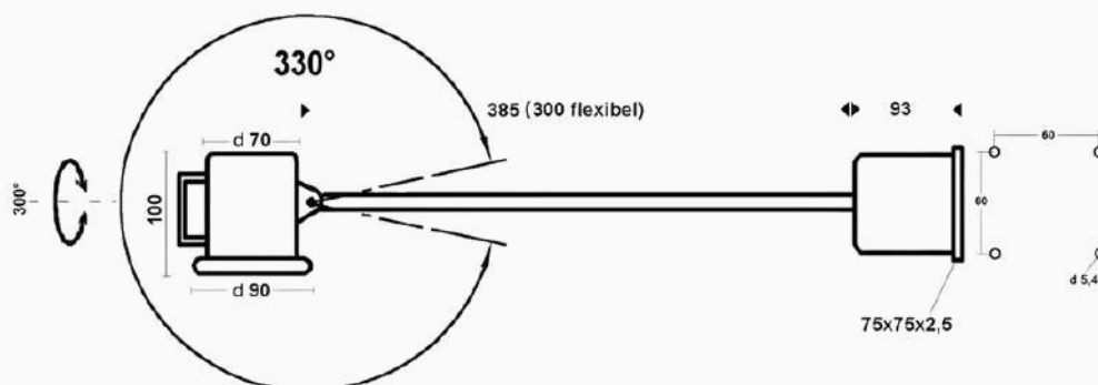
275.90.02-1 (mit Flansch)
