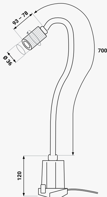
SEITENANSICHT
